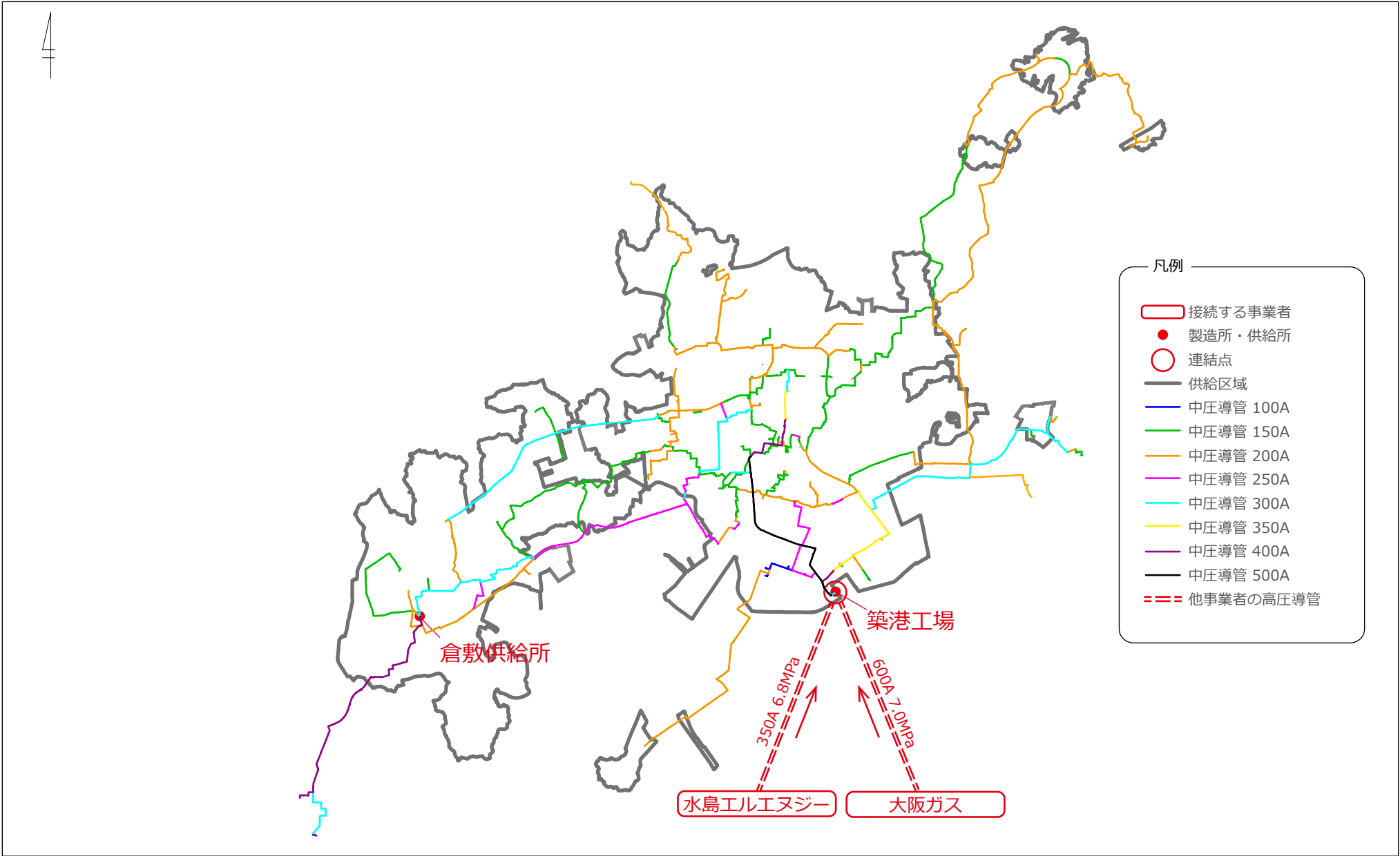
第8表 主要導管図
