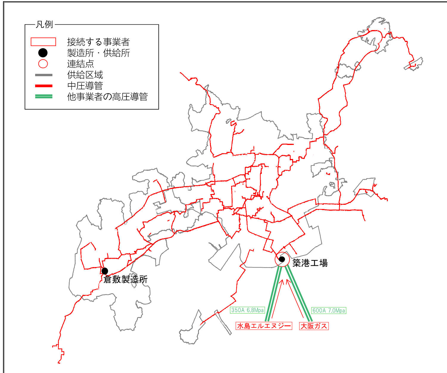
第8表 主要導管図
