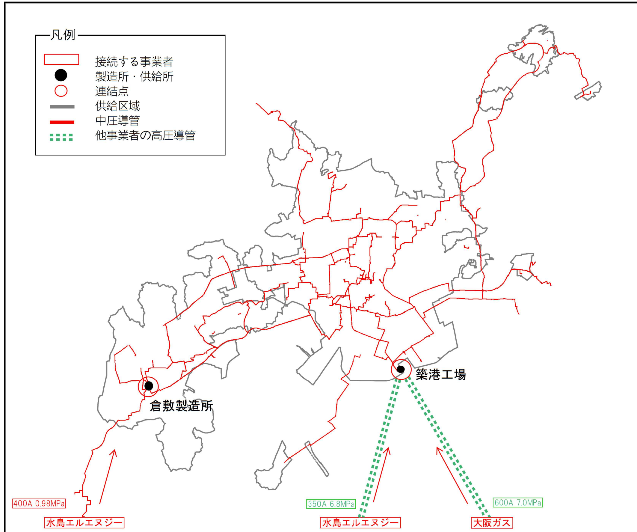
第8表 主要導管図
