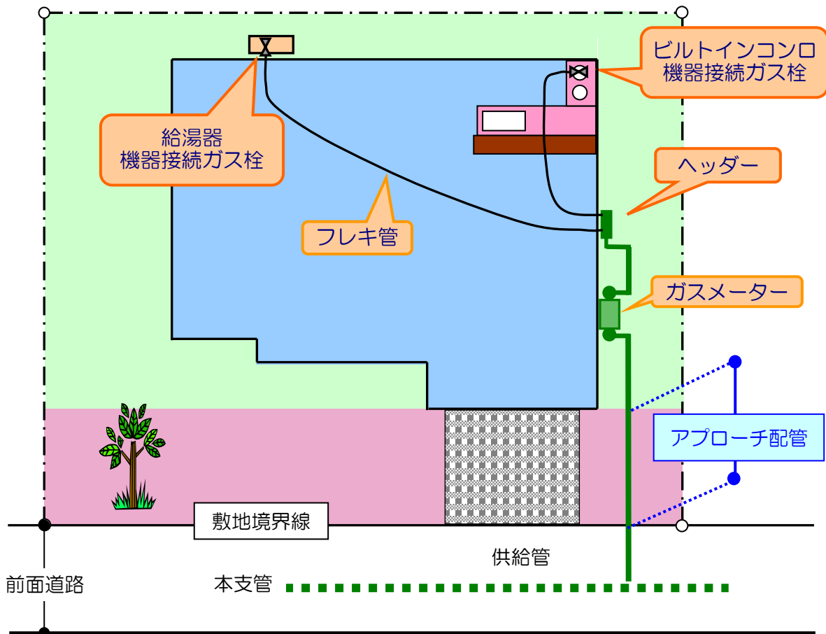
建物標準配管 イメージ図
