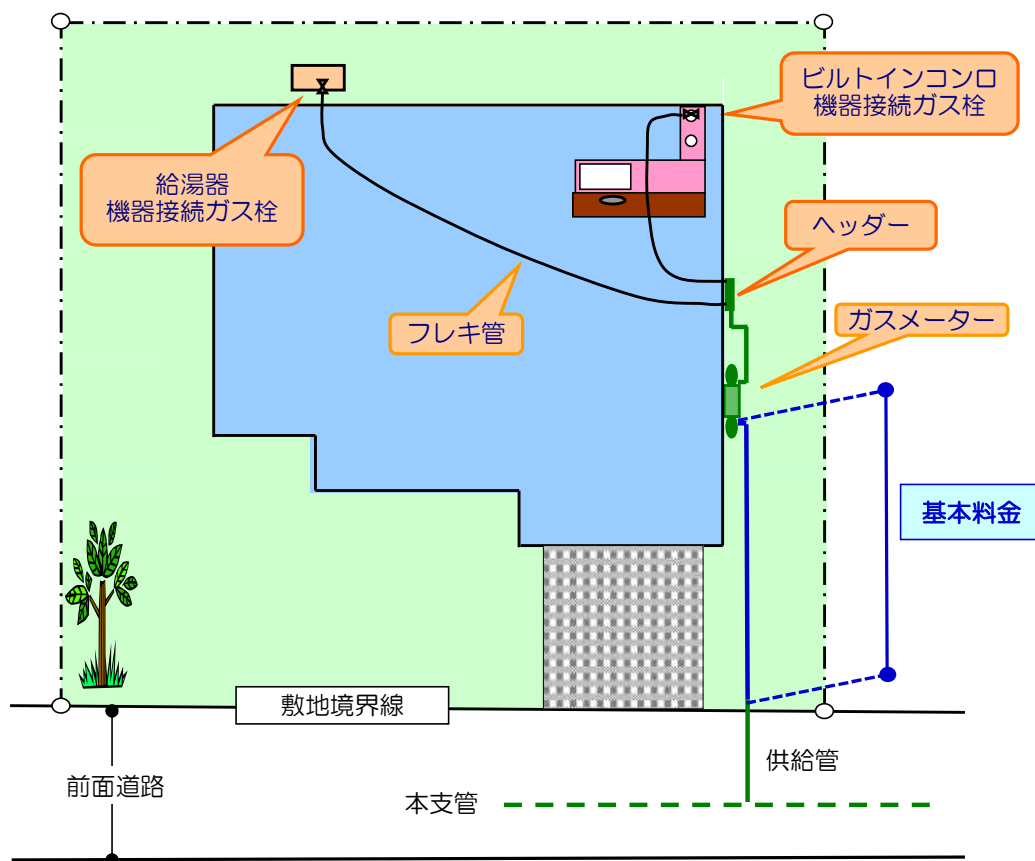
【建物標準配管 イメージ図】
