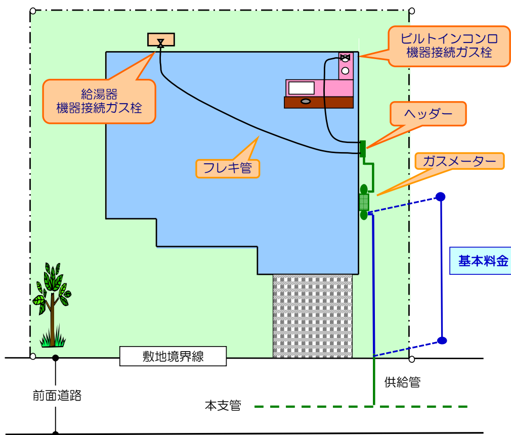
【建物標準配管 イメージ図】
